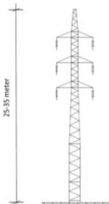
Figur 2. Skiss enbent stål stolpe med vertikalt placerade faslinor.
